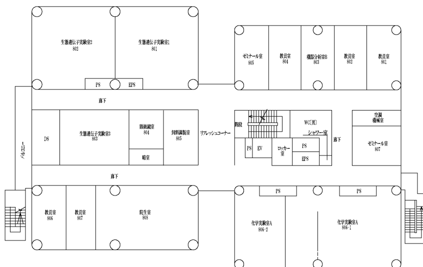
C棟 8階平面図
