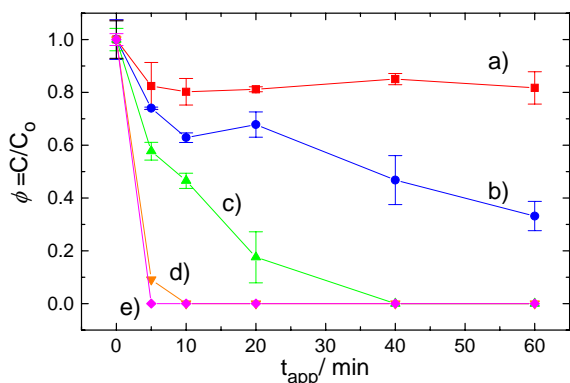
図 7 残存率 vs. t_{app} の E_{app} 依存性 [E2] = 10^{-6} M, 0.1 M Tris, pH 1.0 a) E_{app} = 0 V, b) E_{app} = 0.7 V, c) E_{app} = 0.8 V d) E_{app} = 0.9 V, e) E_{app} = 1.0 V
