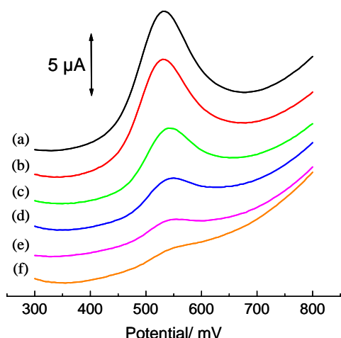
図3 E2 の方形波ボルタモグラム 振幅 25 mV、ステップ電位 5 mV、周波数 5 Hz t_{ac}=5 分 (a) 10 \times 10^{-6} M、(b) 7.5 \times 10^{-6} M、(c) 5.0 \times 10^{-6} M、 (d) 2.5 \times 10^{-6} M、(e) 1.0 \times 10^{-6} M、(f) 0.5 \times 10^{-6} M
