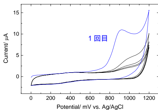
図6 E2 の多重サイクリックボルタモグラム [E2] = 5 mM、0.1 M KCl、pH 1、 掃引速度 0.05 \text{ V s}^{-1} 作用電極：GC 電極 (直径 3 mm)
