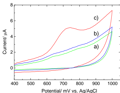
図4 EtBr のサイクリックボルタモグラム [EtBr] = 10^{-4} M、0.1 M Tris、pH 7、 掃引速度 0.1 Vs^{-1} a) 透析膜 GC 電極 b) アルギン酸-透析膜 GC 電極 c) DNA-アルギン酸-透析膜 GC 電極
