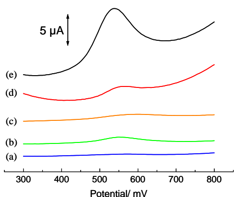
図2 E2 の方形波ボルタモグラム 振幅 25 mV、ステップ電位 5 mV、周波数 5 Hz (a) 未修飾 GC 電極、 t_{ac}=0 (b) 未修飾 GC 電極、 t_{ac}=5 分 (c) Nafion 修飾 GC 電極、 t_{ac}=5 分 (d) MWNT 修飾 GC 電極、 t_{ac}=0 (e) MWNT 修飾 GC 電極、 t_{ac}=5 分
